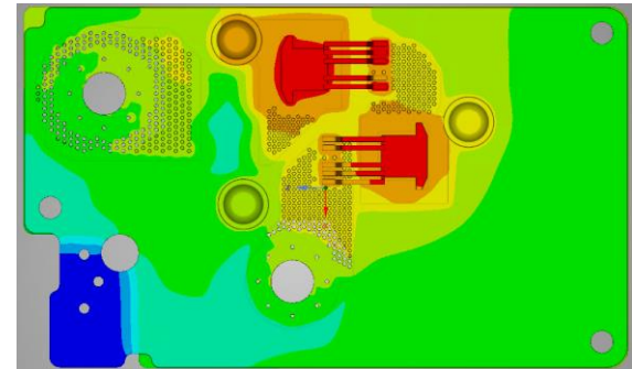
Temperaturausbreitung in der Leistungselektronik
